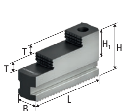
GST Tvrdé stupňovité monoblokové čelisti
