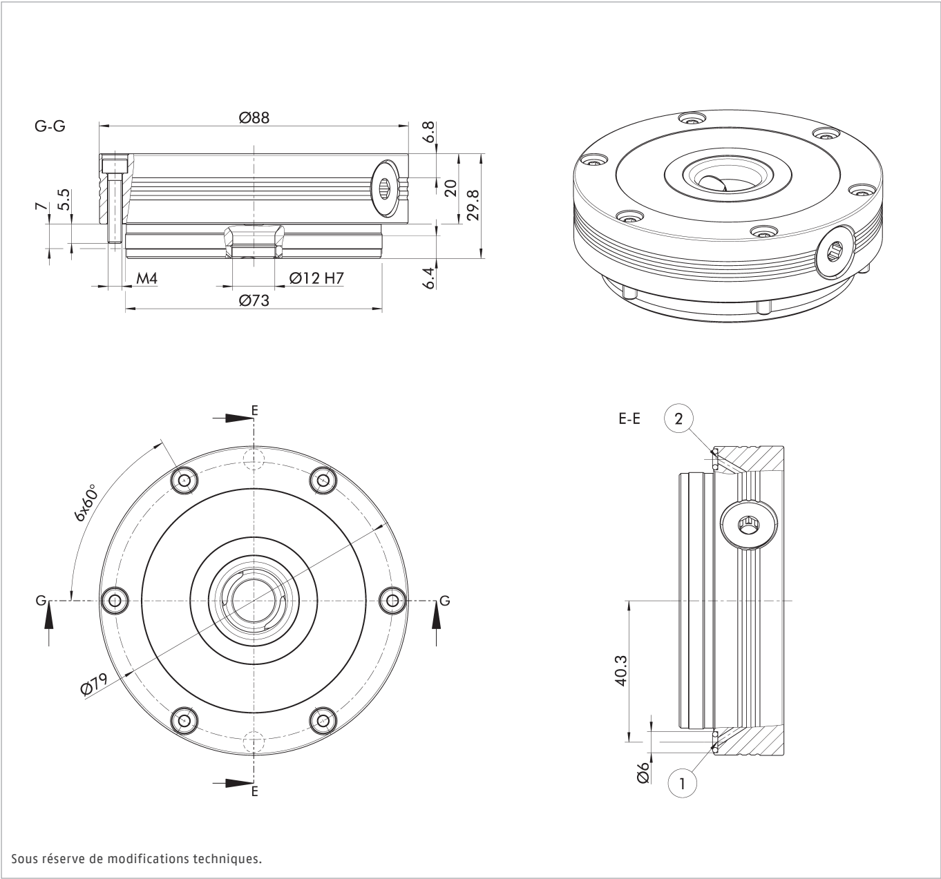
① Raccord direct sans flexible, module ouvert
