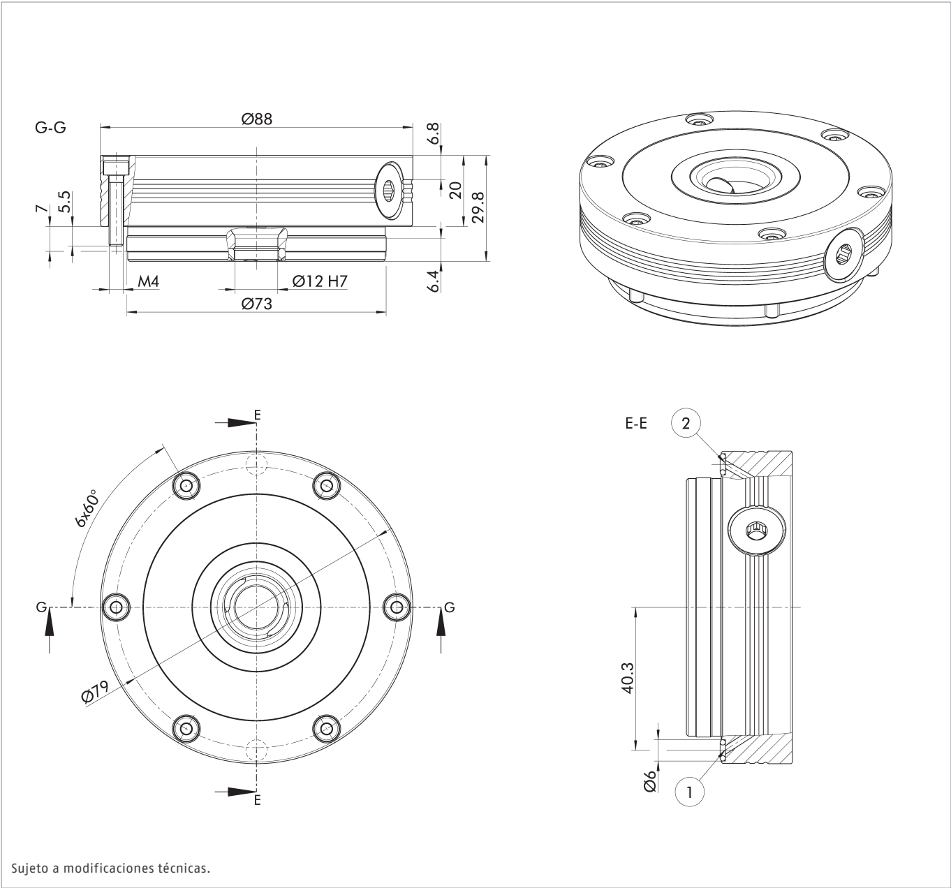
① Módulo abierto con conexión directa sin tubos
