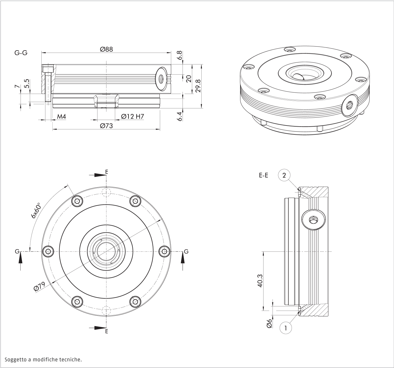
① Collegamento diretto senza tubo flessibile, apertura modulo
