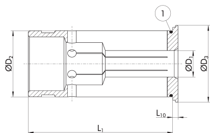
① Těsnění O-kroužku
