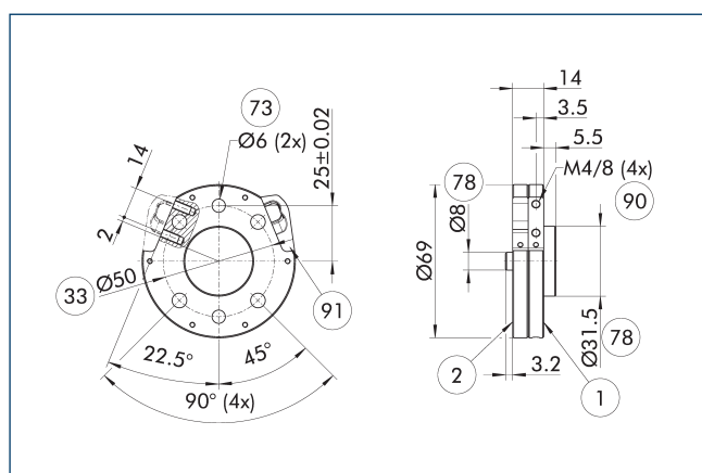
Placa adaptadora A-IS0050/FTS056
