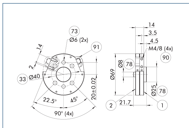
Placa adaptadora A-IS0040/FTS056
