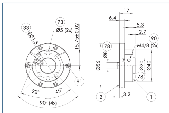
Placa adaptadora A-IS0031/FTS056
