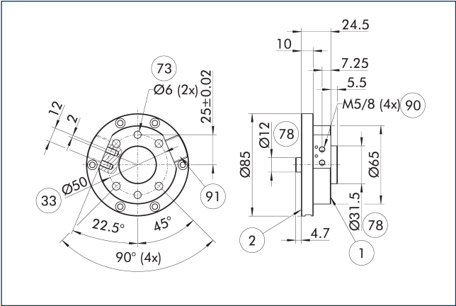
法兰 A-IS0050/FTS085
