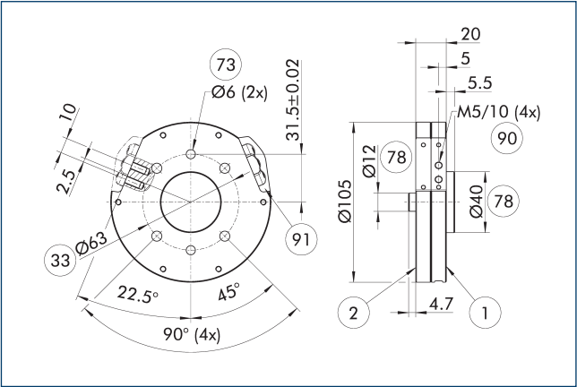
法兰 A-IS0063/FTS085
