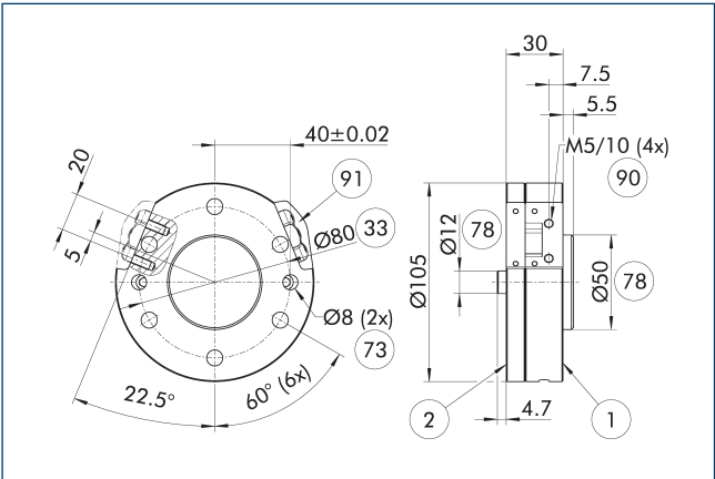
法兰 A-IS0080/FTS085
