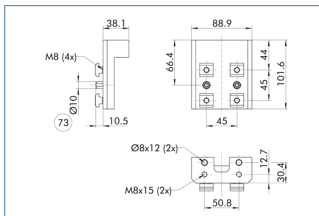
Bloc de fixation CTS C-MB
