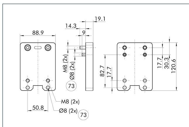
Adaptateur d'extension CTS C-ME
