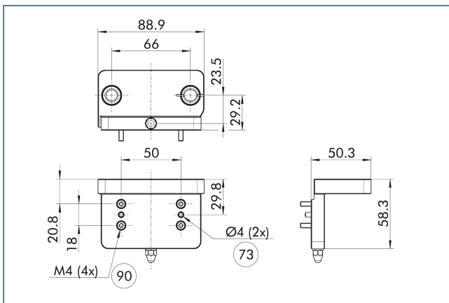
어댑터 플레이트 CTS P-050-AV-J
