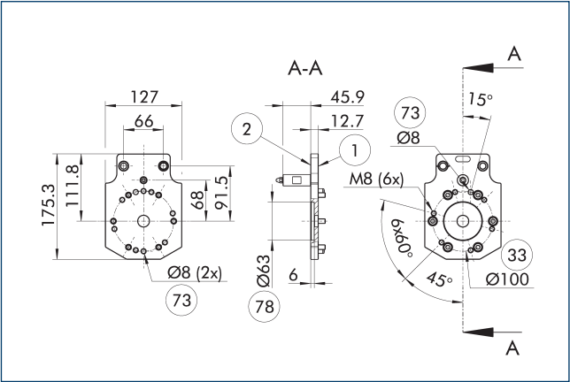
法兰 CTS P-050-AH-CPS046/ISO100
