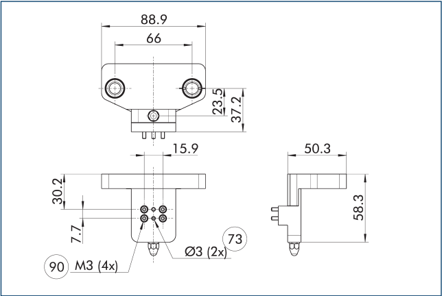
转接板 CTS P-050-AV-S7
