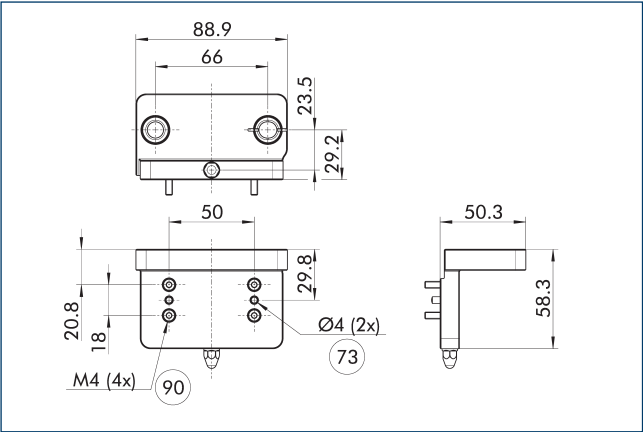
转接板 CTS P-050-AV-J
