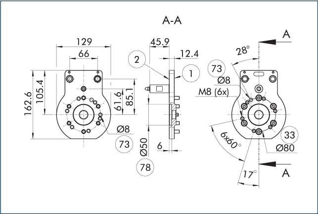
法兰 CTS P-050-AH-CPS041/ISO080
