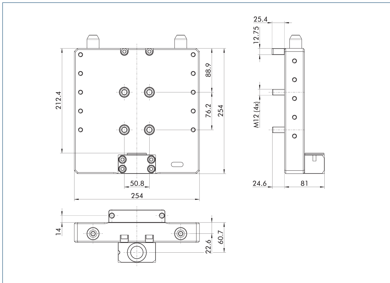
Главный вид CTS P-500-MM
