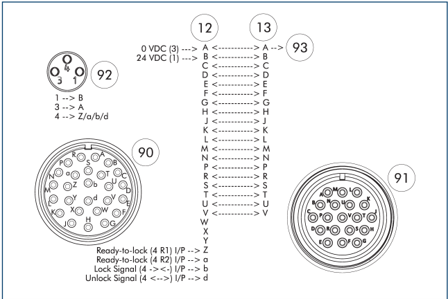
12 Lado del cabezal 13 Lado del adaptador 91 Conector hembra de tapa roscada MS Amphenol, 19 polos 90 Conector macho de tapa roscada MS Amphenol, 26 polos 92 Conector hembra M8, con codificación A, 3 polos 93 perno guía
