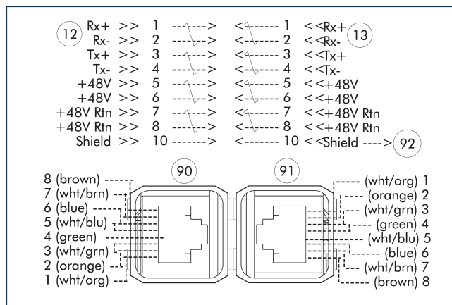
12 Strona urządzenia głównego 91 AIDA PushPull-RJ45 13 Strona adaptera 92 pin prowadzący 90 AIDA PushPull-RJ45
