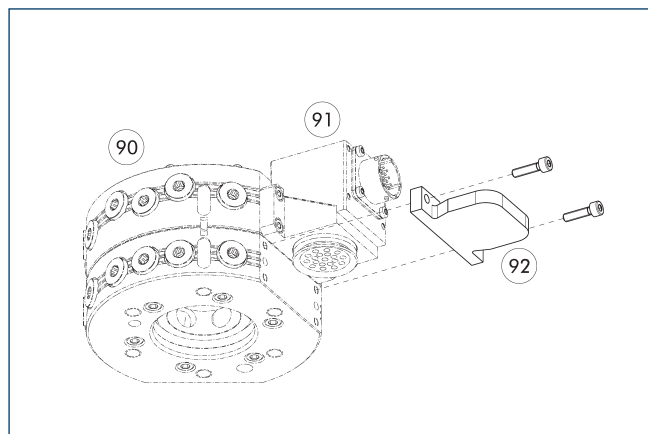
90 Automatyczne zmieniarzki narzędzi CPS 91 Opcjonalny moduł COS master 92 Ośłona COS JPC-A
