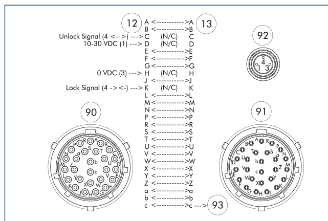
12 Strona urządzenia głównego 91 Gniazdo z blokadą bagietową 13 Strona adaptera Amphenol PT, 26-pinowe 90 Złącze z blokadą bagietową 92 Gniazdo M8, kod A, 3-pinowe Amphenol PT, 26-pinowe 93 pin prowadzący
