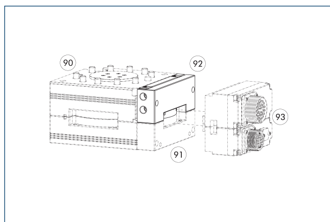
90 Automatyka zmieniająca narzędzi CPS 92 Moduł sterowania pneumatycznego COS master 91 Płyta dystansowa 93 Opcjonalny moduł COS master i adapter
