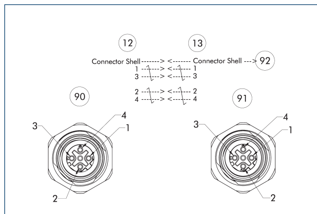
12 Strona urządzenia głównego 91 M12, złącze żeńskie kodowanie D 13 Strona adaptera 92 pin prowadzący 90 M12, złącze żeńskie kodowanie D
