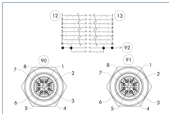
12 Strona urządzenia głównego 91 Gniazdo M12, kod X 13 Strona adaptera 92 pin prowadzący 90 Gniazdo M12, kod X
