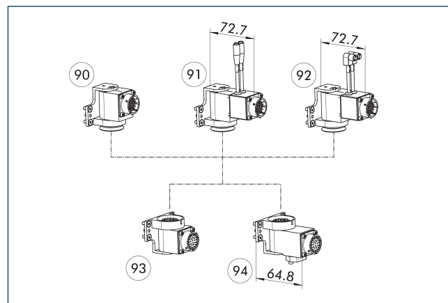
90 COS G26-K 91 COS G26W-K 92 COS G26R-K
