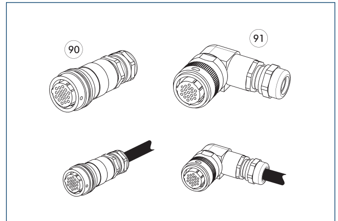
⑨② 플러그/소켓 스트레이트
