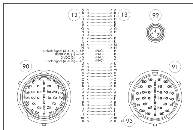
⑨1 Amphenol PT 바요넷 록 소켓, 36핀
