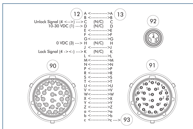
12 Strona urządzenia głównego 91 Gniazdo z blokadą bagietową Amphenol PT, 26-pinowe 13 Strona adaptera 92 Gniazdo M8, kod A, 3-pinowe 90 Złącze z blokadą bagietową Amphenol PT, 26-pinowe 93 pin prowadzący
