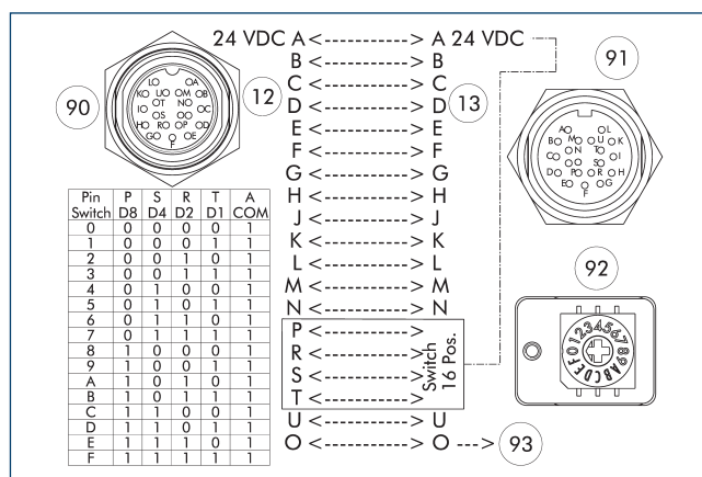
12 Strona urządzenia głównego 91 Gniazdo M16, 19-pinowe 13 Strona adaptera 92 Przetłącznik obrotowy enkodera do kodowania do 15 narzędzi. 90 Złącze M16, 19-pinowe 93 pin prowadzący
