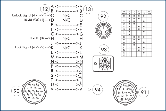
12 Ведущая сторона 13 Переходная сторона 90 Разъем Amphenol PT с байонетным замком, 19 контактов 91 Гнездо Amphenol PT с байонетным замком, 19 контактов 92 Гнездо M8, маркировка A, 3 контакта 93 Поворотный переключатель для кодировки от 0 до 15 инструментов. 94 опережающий штифт
