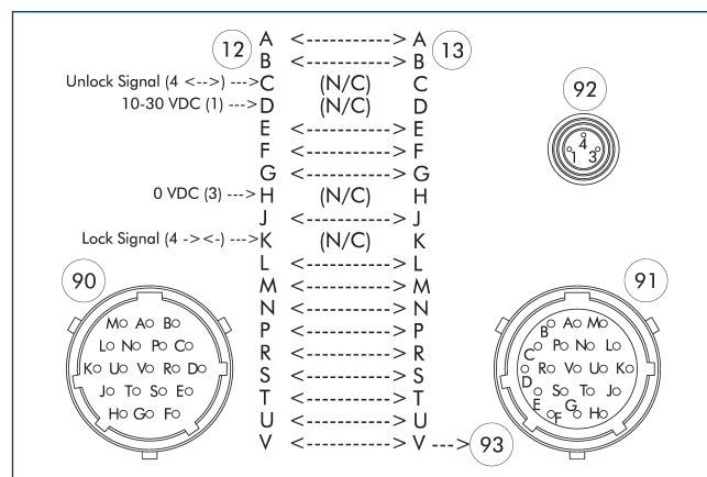
COS R19W-K 和 COS R19-A 的引脚分配
