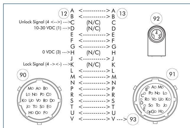
COS R19R-K 和 COS R19-A 的引脚分配
