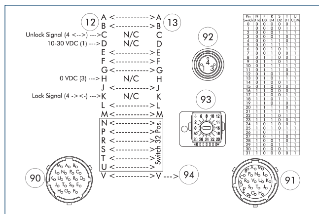
COS R19W-K 和 COS R13-A 的引脚分配
