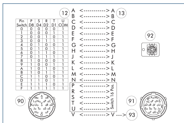
COS R19-K 和 COS R14-A 的引脚分配
