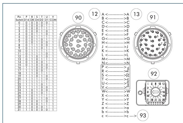
12 Strona urządzenia głównego 91 Gniazdo z blokadą bagnetową Amphenol PT, 26-pinowe 13 Strona adaptera 92 Przetątnik obrotowy enkodera do kodowania narzędzi obsługujący do 31 narzędzi. 90 Złącze z blokadą bagnetową Amphenol PT, 26-pinowe 93 pin prowadzący
