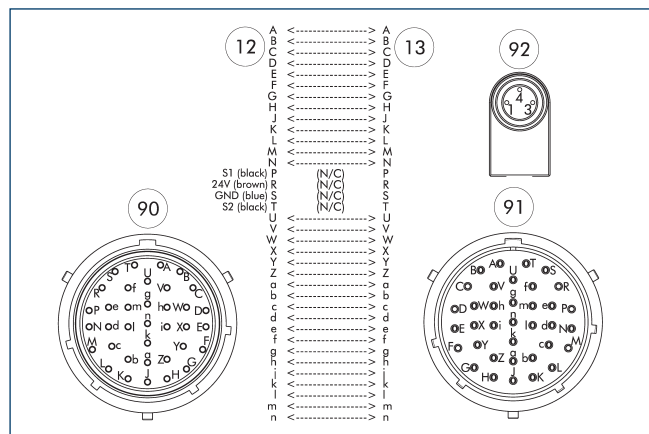
12 Strona urządzenia głównego 91 Gniazdo z blokadą bagnetową 13 Strona adaptera Amphenol PT, 36-pinowe 90 Złącze z blokadą bagnetową 92 Gniazdo M8, kod A, 3-pinowe Amphenol PT, 36-pinowe 93 pin prowadzący
