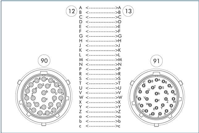
12 Strona urządzenia głównego 13 Strona adaptera 90 Złącze z blokadą bagietową Amphenol PT, 26-pinowe 91 Gniazdo z blokadą bagietową Amphenol PT, 26-pinowe
