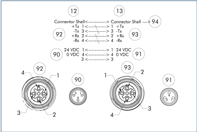
12 Lado del cabezal 92 Conector hembra con codificación D M12 13 Lado del adaptador 93 Conector hembra con codificación D M12 90 Conector macho M8, con codificación A, 3 polos 94 perno guía 91 Conector hembra M8, con codificación A, 3 polos
