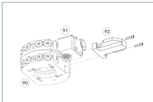
90 Automatyczne zmieniarki narzędzi CPS 91 Opcjonalny moduł COS master 92 Ostona COS KPC-A
