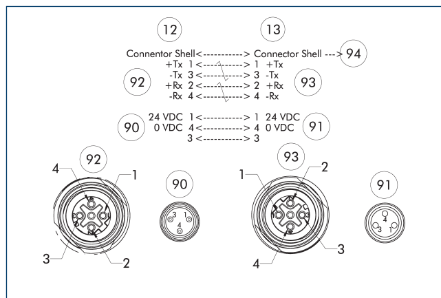
12 Strona urządzenia głównego 92 M12, złącze żeńskie kodowanie D 13 Strona adaptera 93 M12, złącze żeńskie kodowanie D 90 Złącze M8, kod A, 3-pinowe 94 pin prowadzący 91 Gniazdo M8, kod A, 3-pinowe
