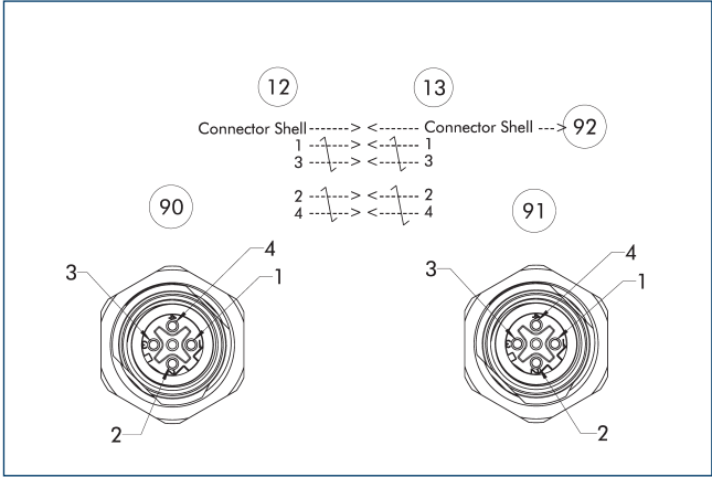
12 Ведущая сторона 13 Переходная сторона 90 Гнездо M12 с ключом «D» 91 Гнездо M12 с ключом «D» 92 опережающий штифт
