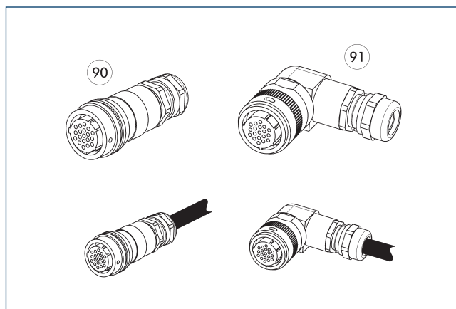
90 Zástrčka/zdírka přímá
