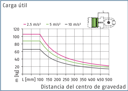
Diagrama de carga – diseño horizontal
