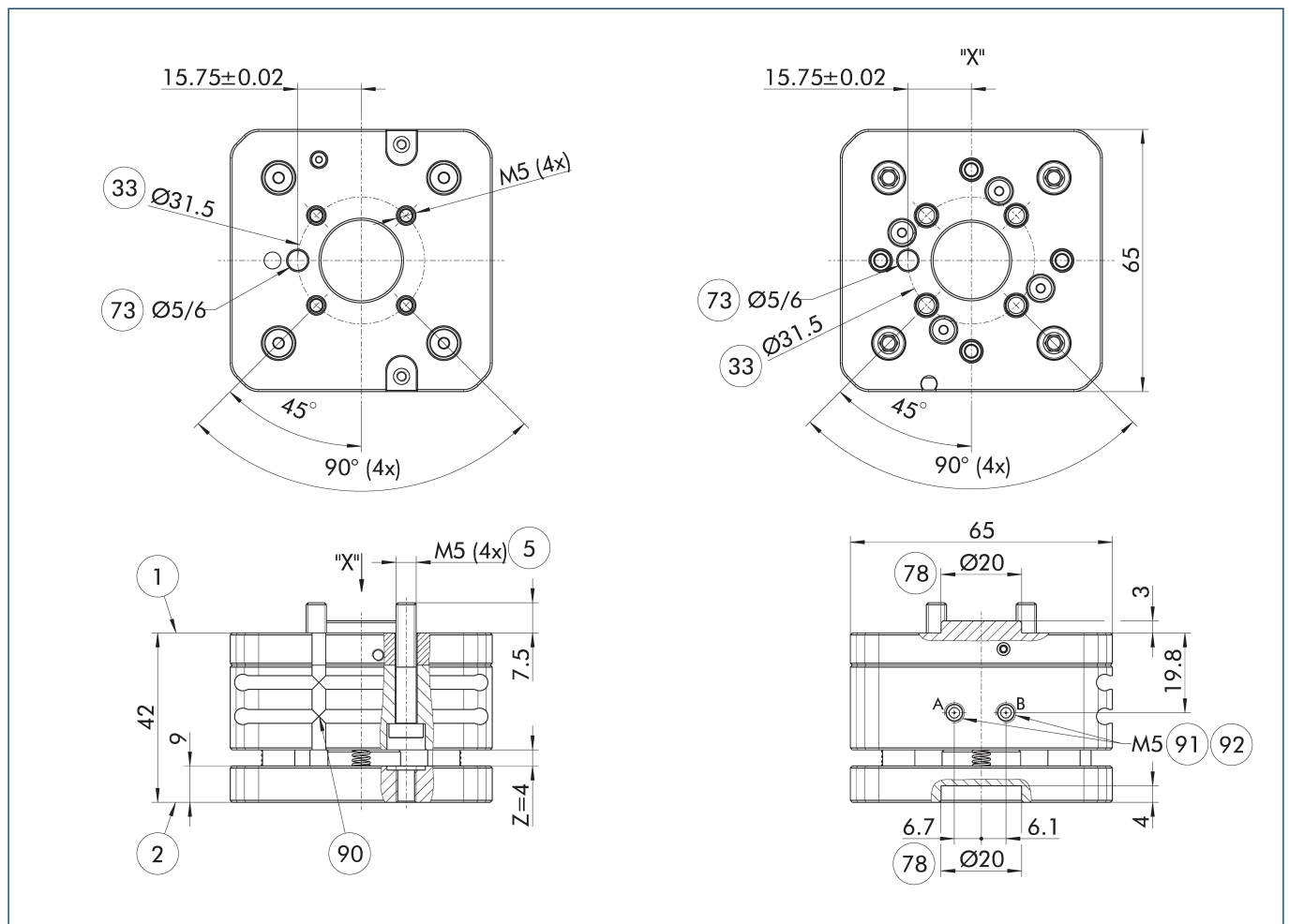
主视图 AGM-Z 031
