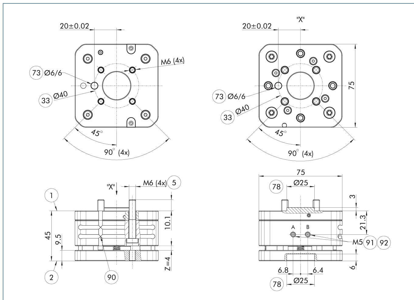
主视图 AGM-Z 040
