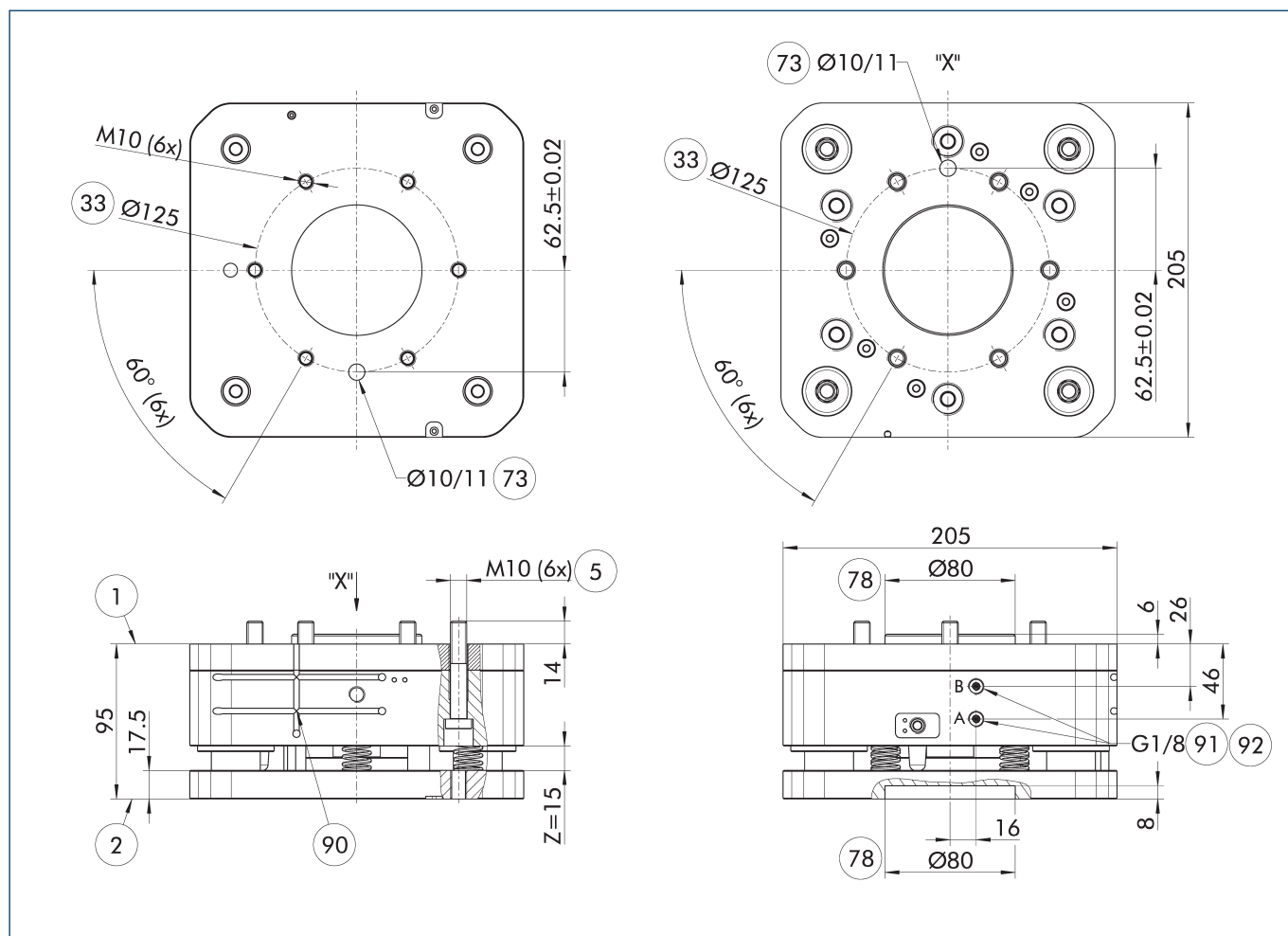
主视图 AGM-Z 125
