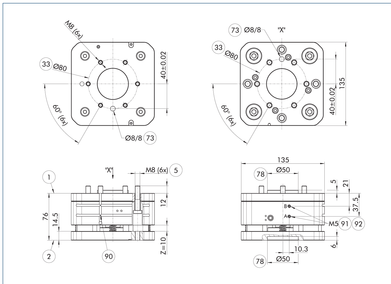
主视图 AGM-Z 080
