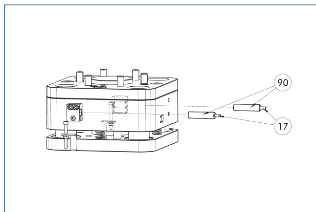
17 Кабельный выход 90 Бесконтактный датчик IN
