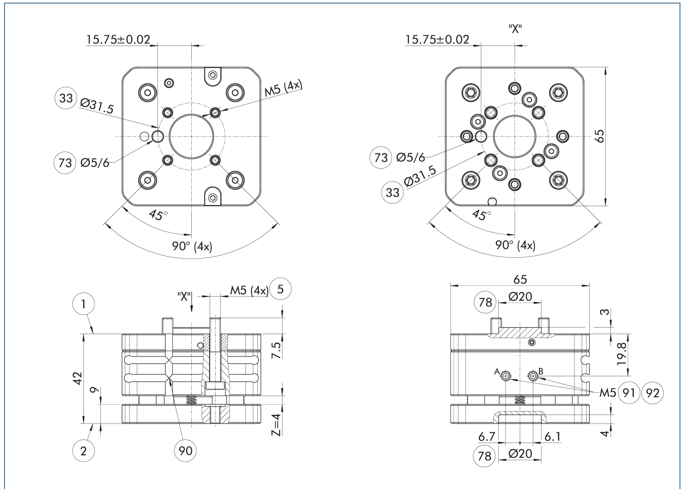
主视图 AGM-Z 031
