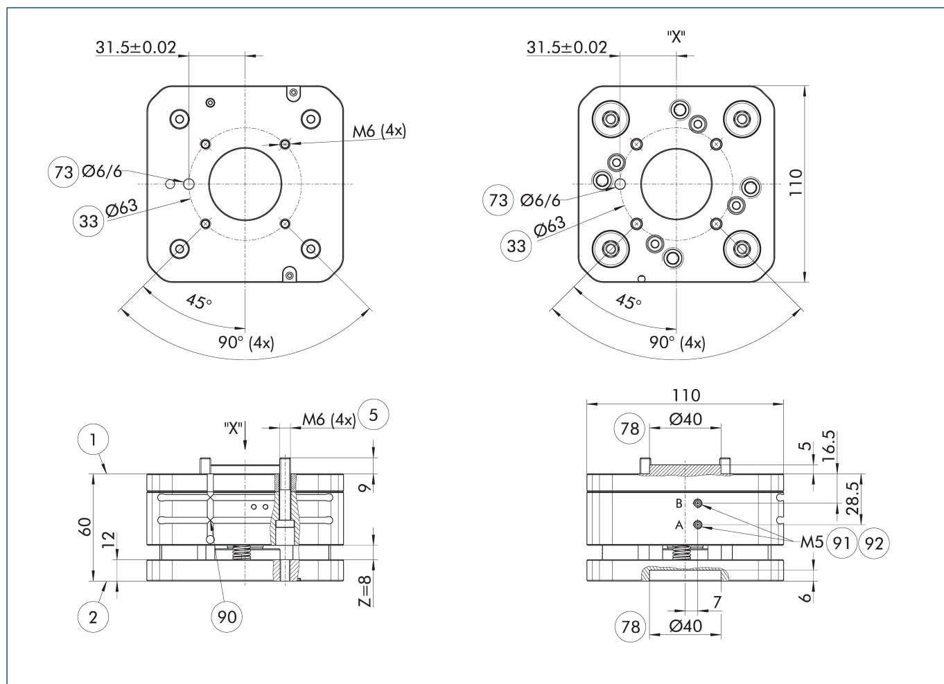
主视图 AGM-Z 063
