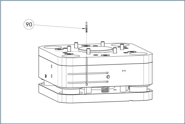
90 传感器 MMS 22...-PI2...
