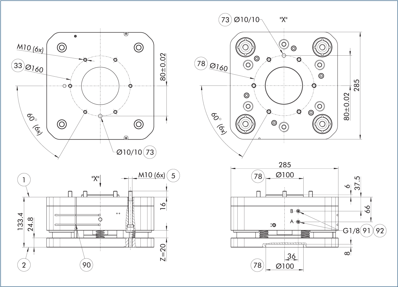
主视图 AGM-Z 160L
