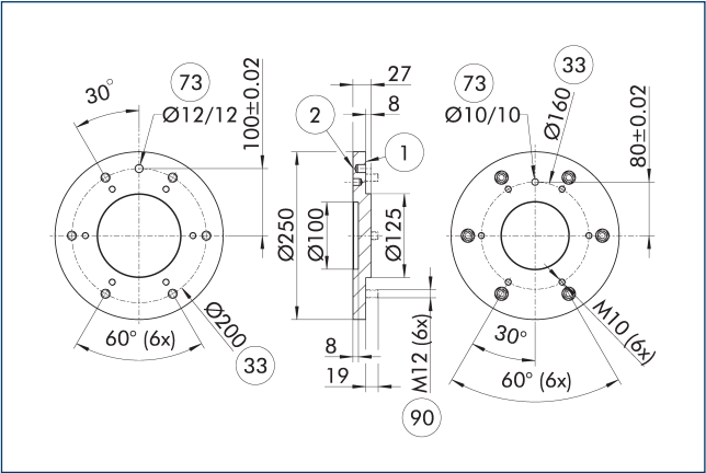
法兰 A-IS0160/ISO200
