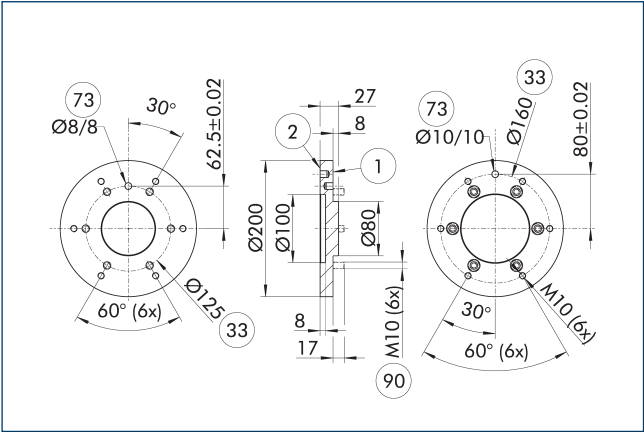
法兰 A-IS0160/ISO125
