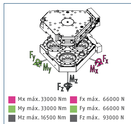
Cargas máx.
