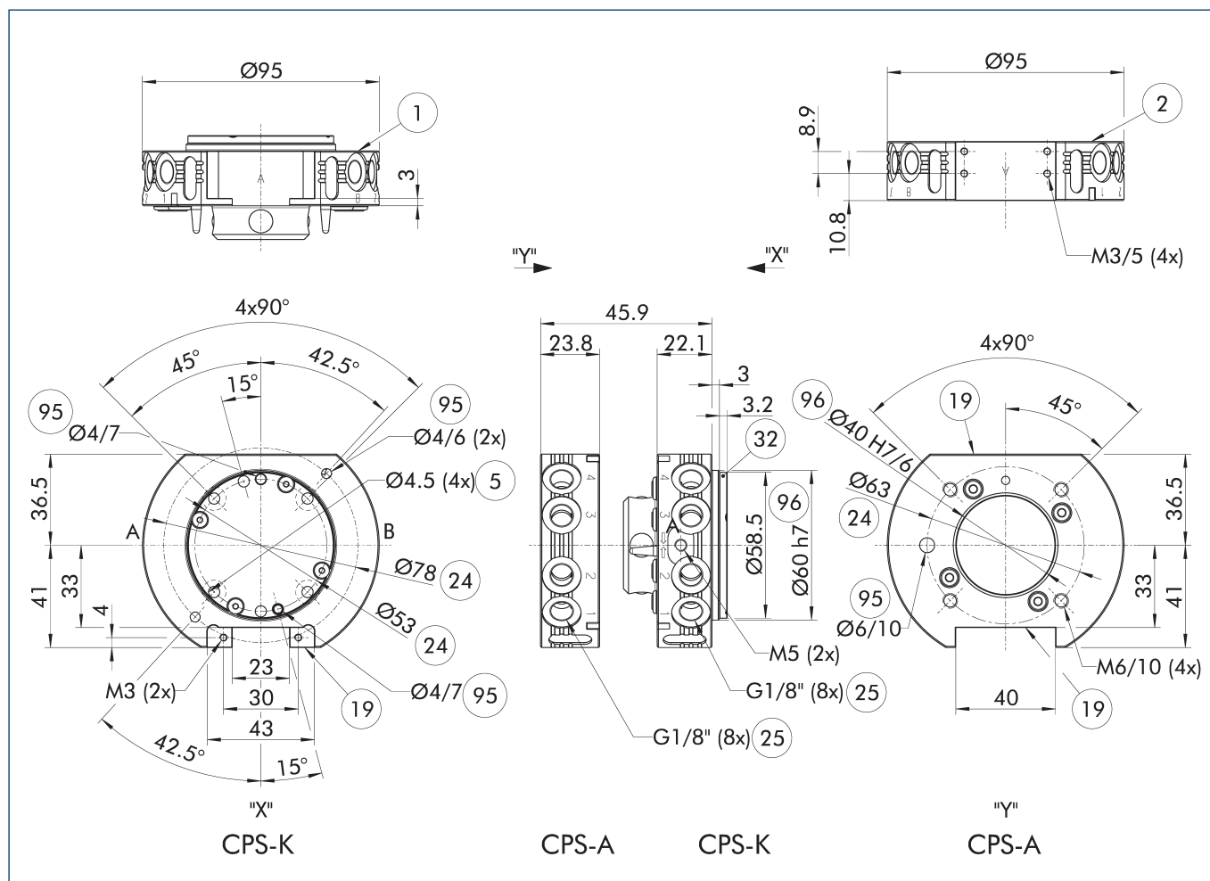
主视图
