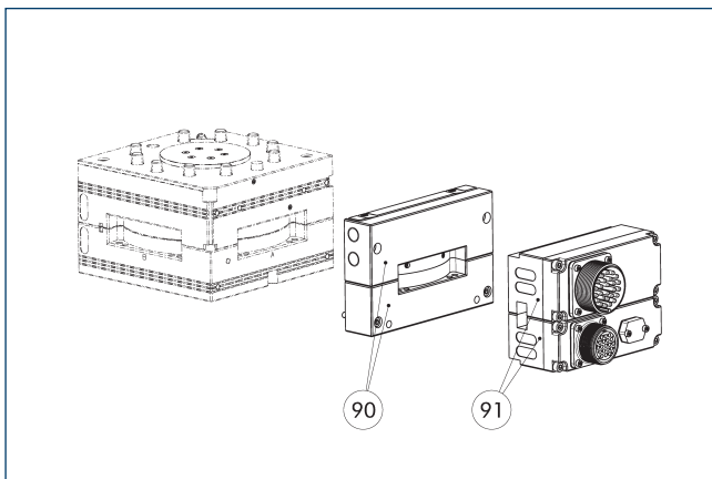
90 공압 제어 모듈 및 스페이스 플레이트
