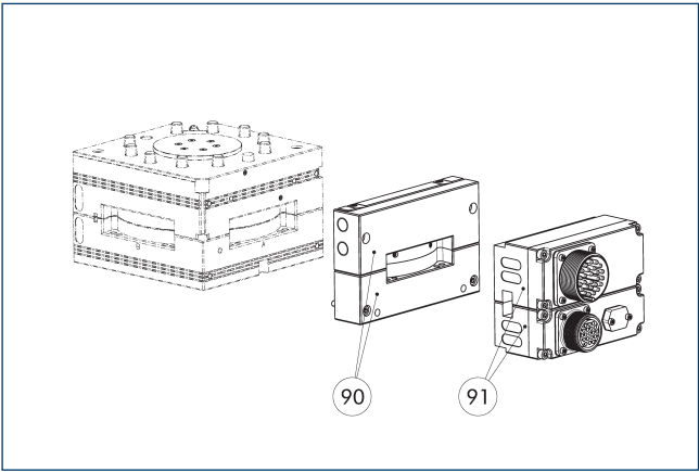
⑨0 Moduł sterowania pneumatycznego i płyta dystansowa ⑨1 Moduł opcjonalny COS
