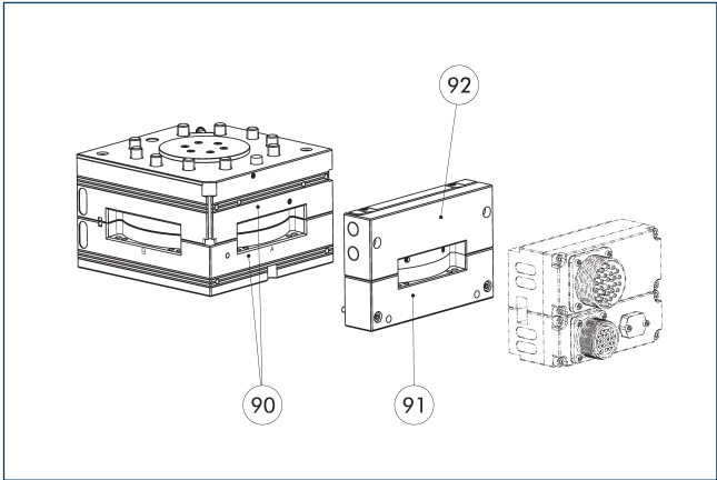
⑨0 Powierzchnia montażowa A dla modułów sterujących ⑨2 Moduł sterowania pneumatycznego ⑨1 Płyta dystansowa
