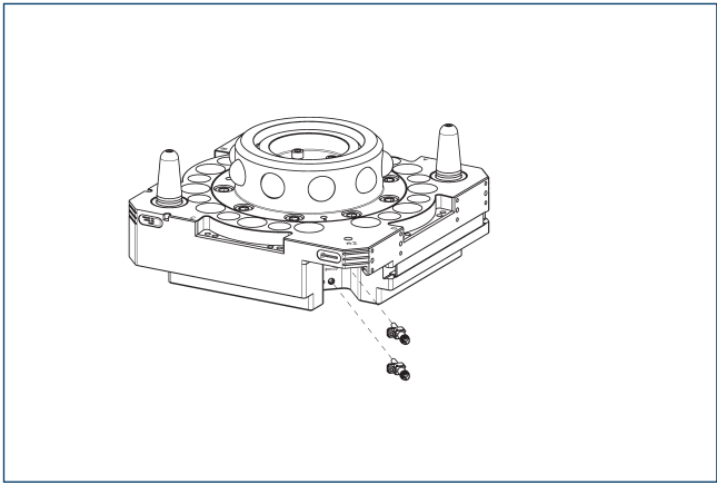
⑨0 Zestaw montażowy do monitorowania blokowania/odblokowywania (uchwyt i czujnik)
