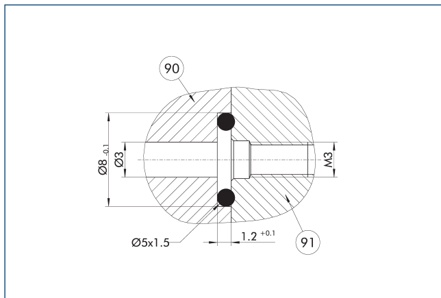
90 어댑터 플레이트
