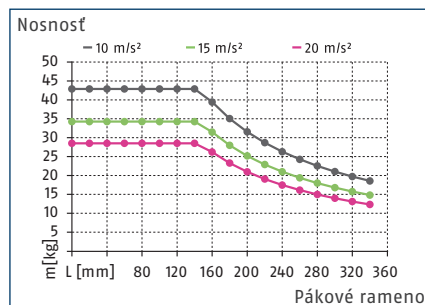
Graf zaťaženia
