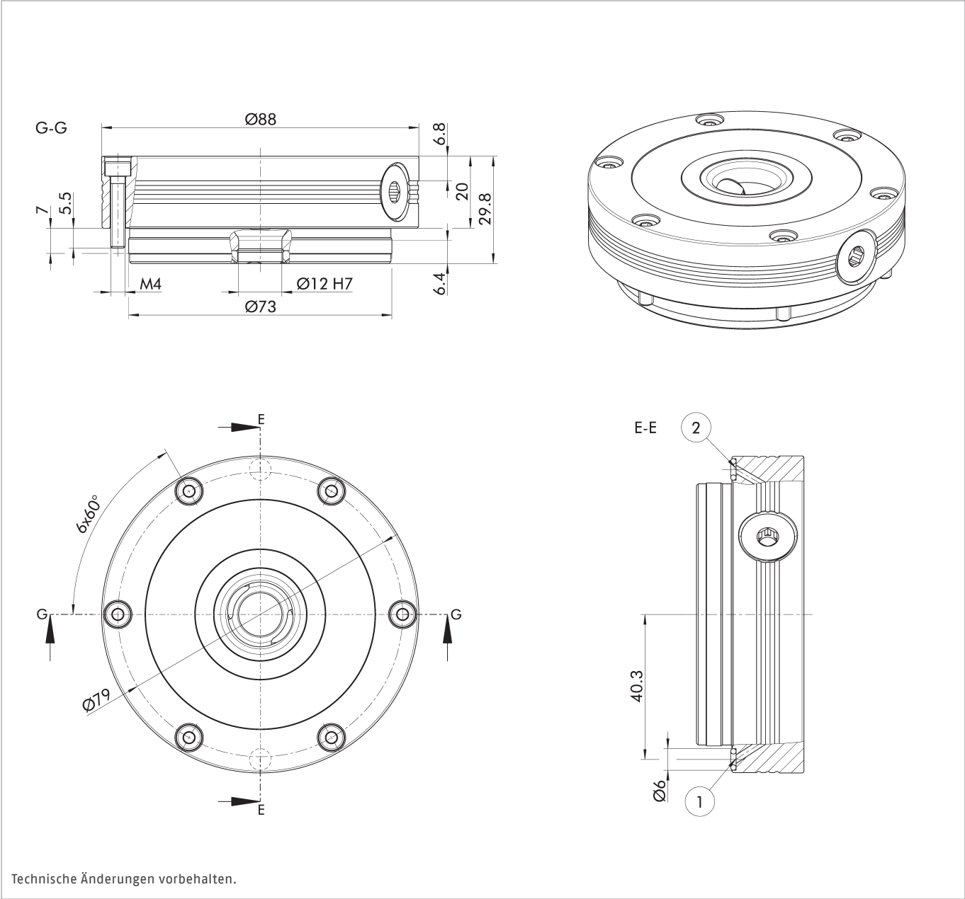
① Schlauchloser Direktanschluss Modul öffnen
