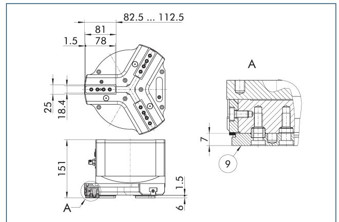
9 장착 나사 연결도를 보려면 기본 버전 참조
