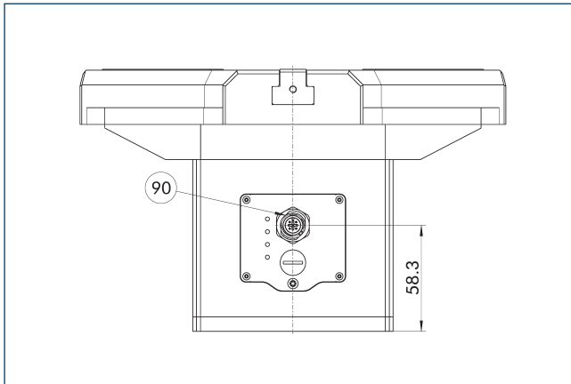
90 전압 공급 및 통신(M12, 커넥터, A-코딩, IL: 5핀, MB: 4핀)
