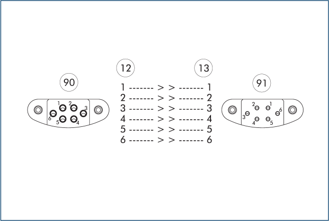
12 Ведущая сторона 90 Паяные контакты 13 Переходная сторона 91 Паяные контакты
