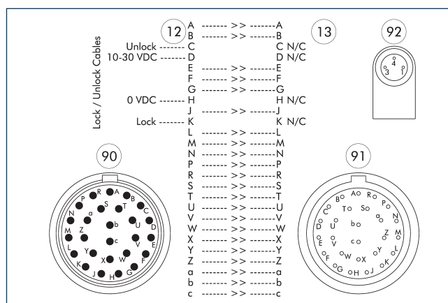
⑫ マスター側 ⑬ アダプター側 ⑨⑩ Amphenol PT バヨネットロック コネクタ, 26 ピン
