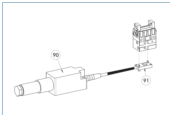
90 Auswerteelektronik FPS-F5
