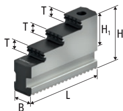
STF Harte Stufenblockbacken
