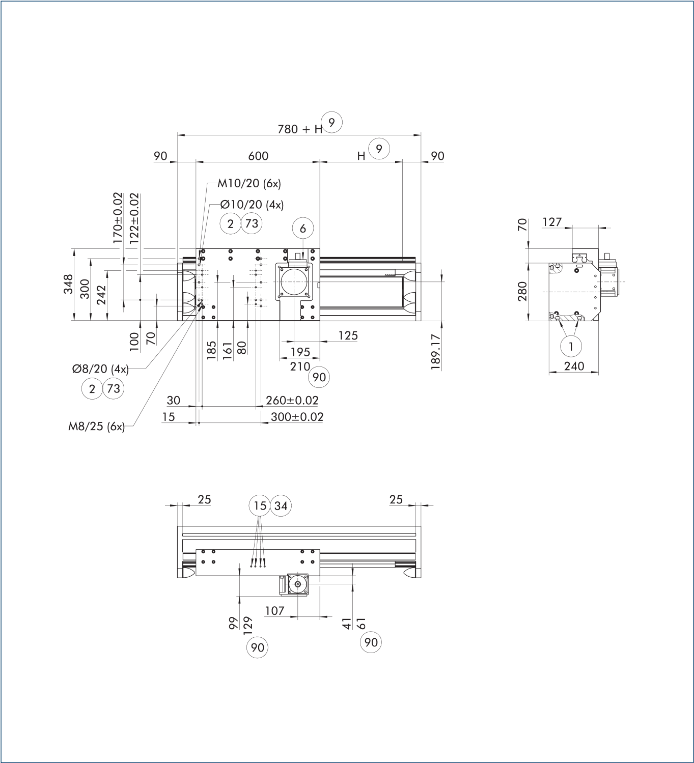
AZSS 主视图
