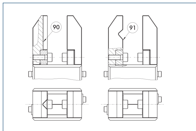
⑨⑩ Prisma disposto verticalmente
