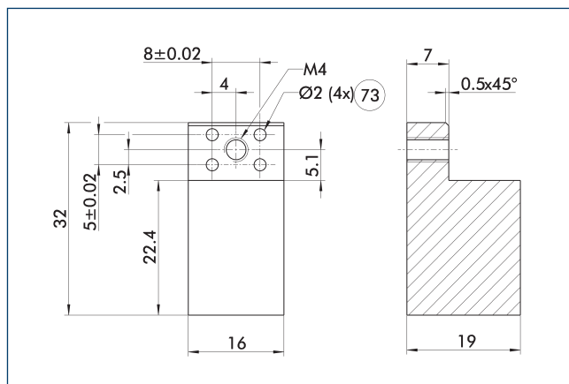
Il disegno mostra la griffa grezza che può essere rialzata a cura del cliente.
