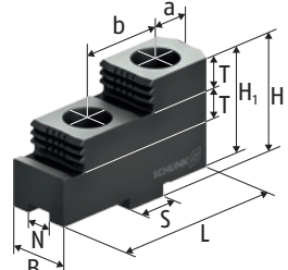
SHF Harte Stufenaufsatzbacken
