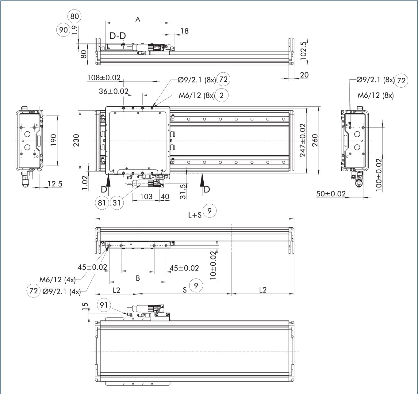
主视图: 单电机版本 (SLD 21)
