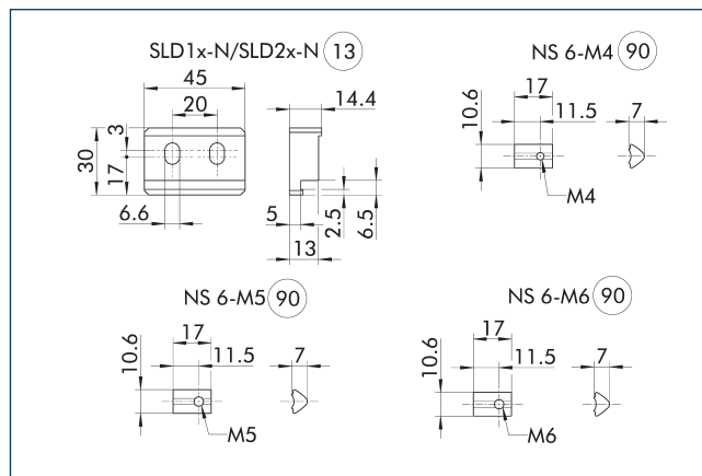
⑬ 安裝帶
