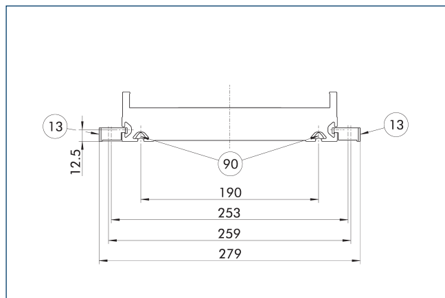
⑬ 安裝帶
