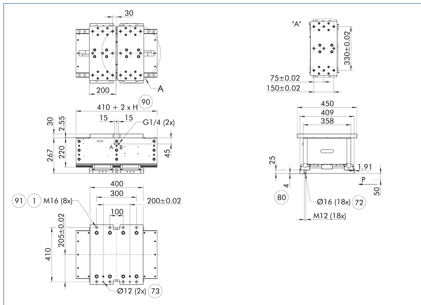
主视图 PLG 120-...-1-...
