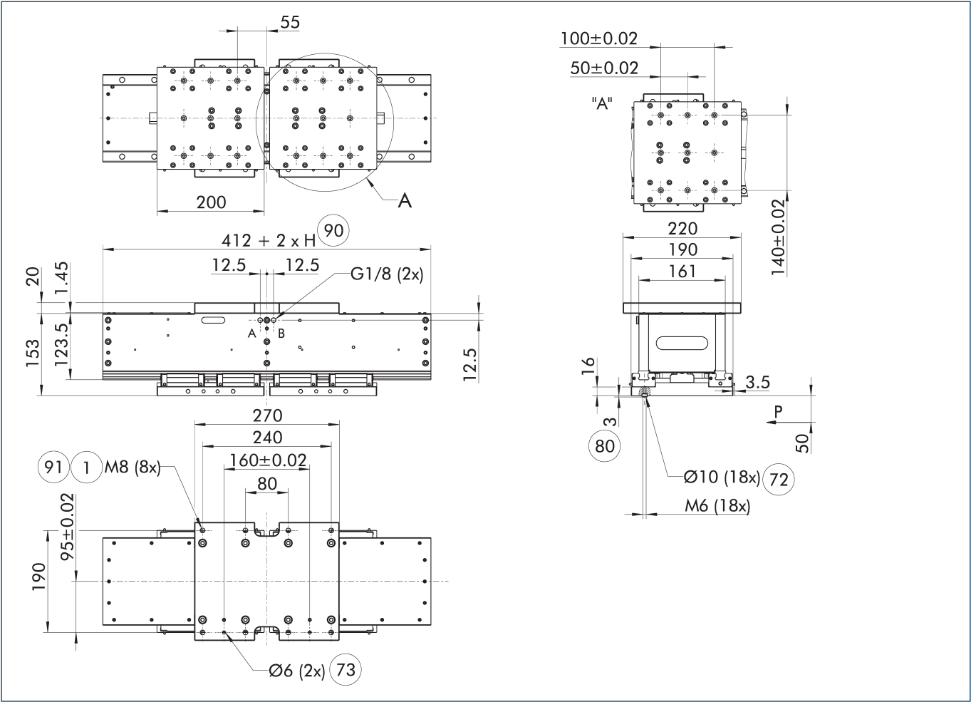
主视图 PLG 20-...-2-...
