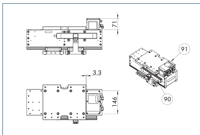
⑨0 Unité de positionnement pneumatique PPD ⑨1 Détecteurs de proximité inductifs
